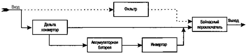
Рис. 2.37. Структурная схема UPS типа line interactive
