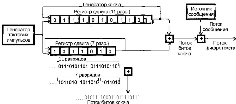
Рис. 4.23. Генератор потокового ключа
