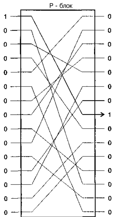
Рис 4.26. Блок перестановок с большим количеством вариантов коммутации
