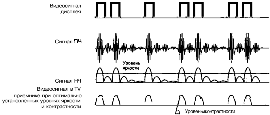
Рис. 2.11. Временные диаграммы сигналов, обрабатываемых ТВ-приемником
