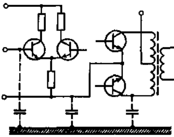
Рис. 2.31. Примеры путей распространения импульсных помех
