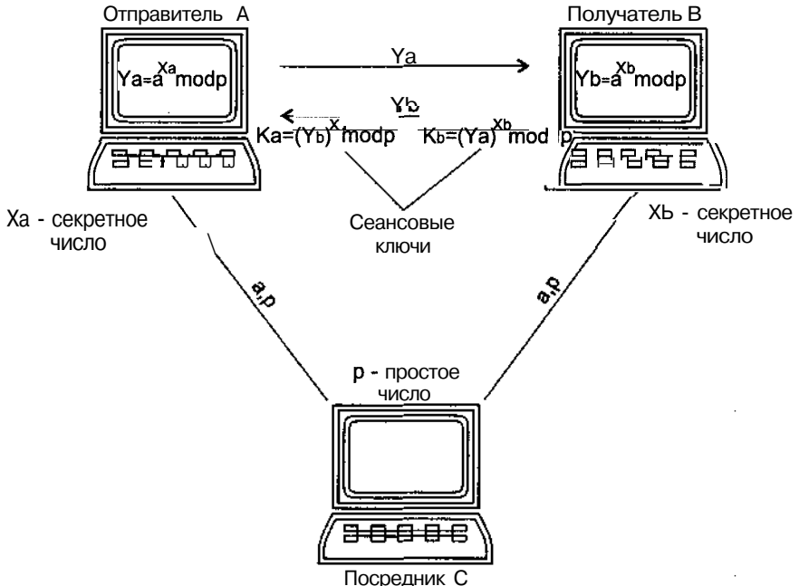
Рис. 4.30. Протокол передачи ключа по незащищенному каналу
