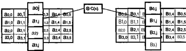
Рис. 4.13. Преобразование замешивания столбцов MixColumn
