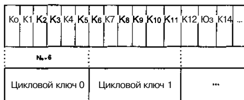
Рис. 4.15. Расширение ключа и выбор циклового ключа
