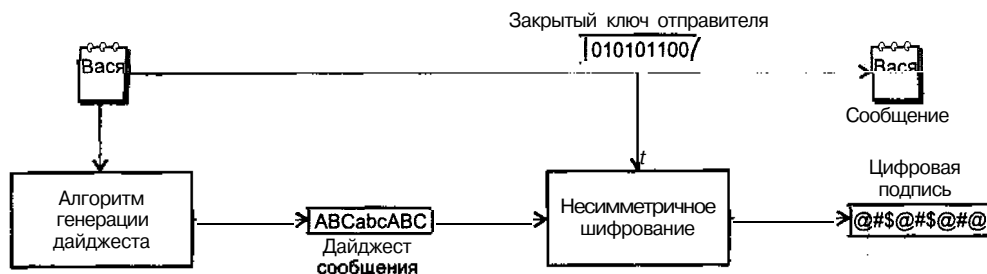
Рис. 4.35. Реализация ЭЦП
