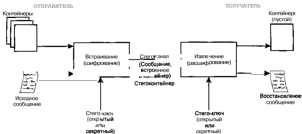
Рис. 5.1. Обобщенная стегосистема
