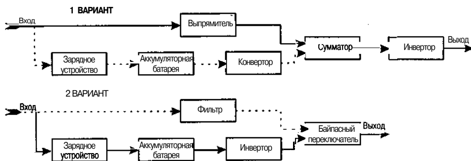
Рис. 2.36. Структурная схема UPS типа on-line
