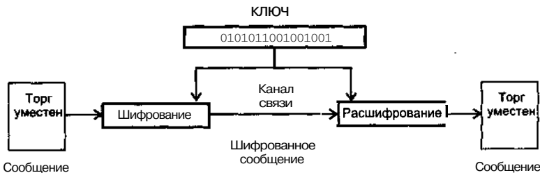
Рис. 4.2. Симметричное шифрование
