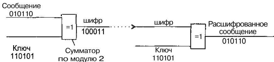
Рис. 4.22. Двоичная подстановка
