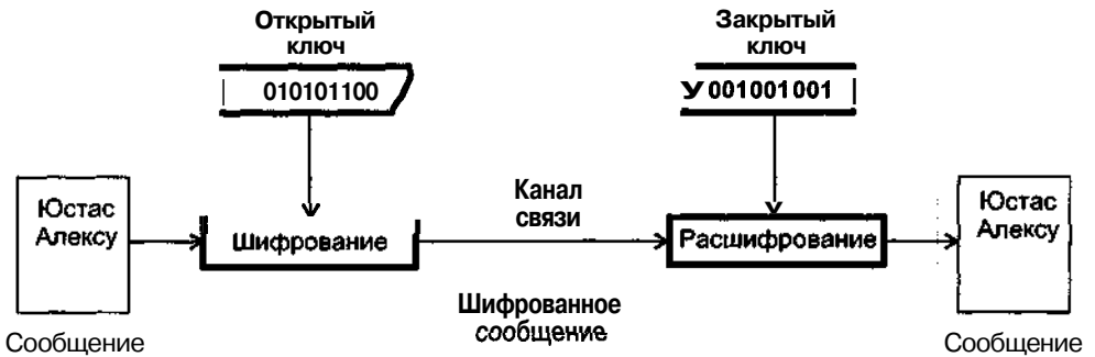
Рис. 4.3. Несимметричное шифрование
