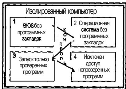
Рис. 3.37. Изолированный компьютер
