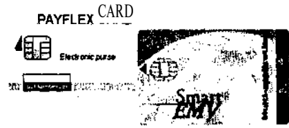
Рис. 3.16. Многоцелевая смарт-карта
