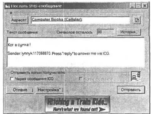
Рис. 7.9. Отправление SMS-сообщения
