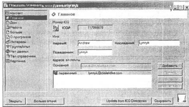
Рис. 3.11. Вкладка Main
